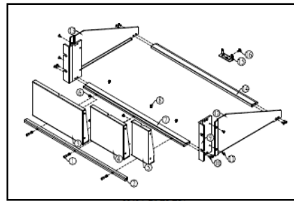
Model 2260B-RMK-EIA: 机架安装套件 (EIA 机架)。
