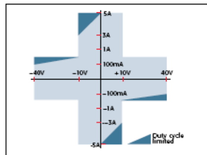
2440型5A源表
