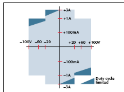
2425型100W源表
