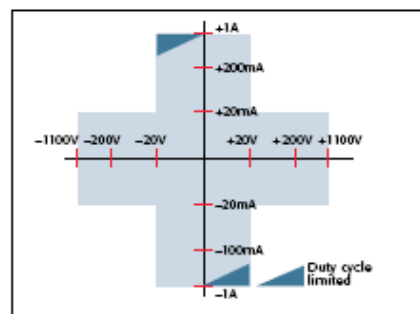
2410型高压源表
