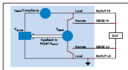
加压, 测量电流、电压或电阻结构
