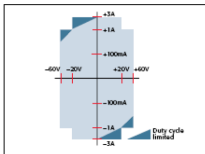
2420型3A源表
