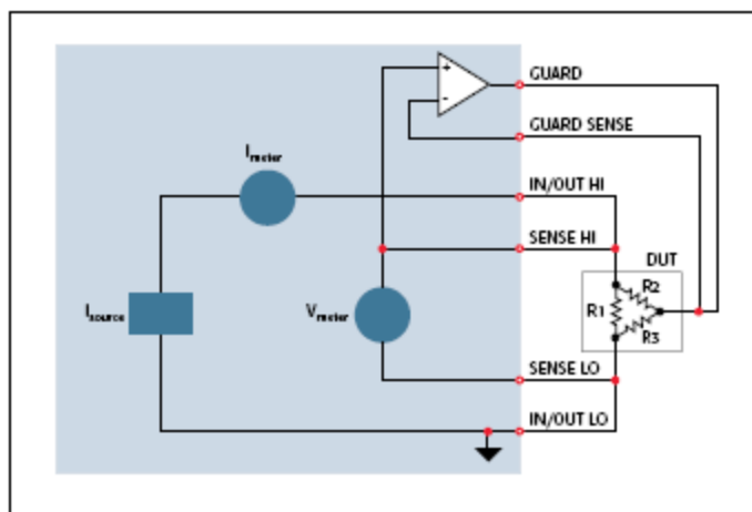
接触检查选项适于4线或6线应用
